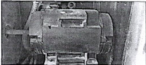
IMÁGENES DE MOTOR 30 HP, CARCASA 180 L.
