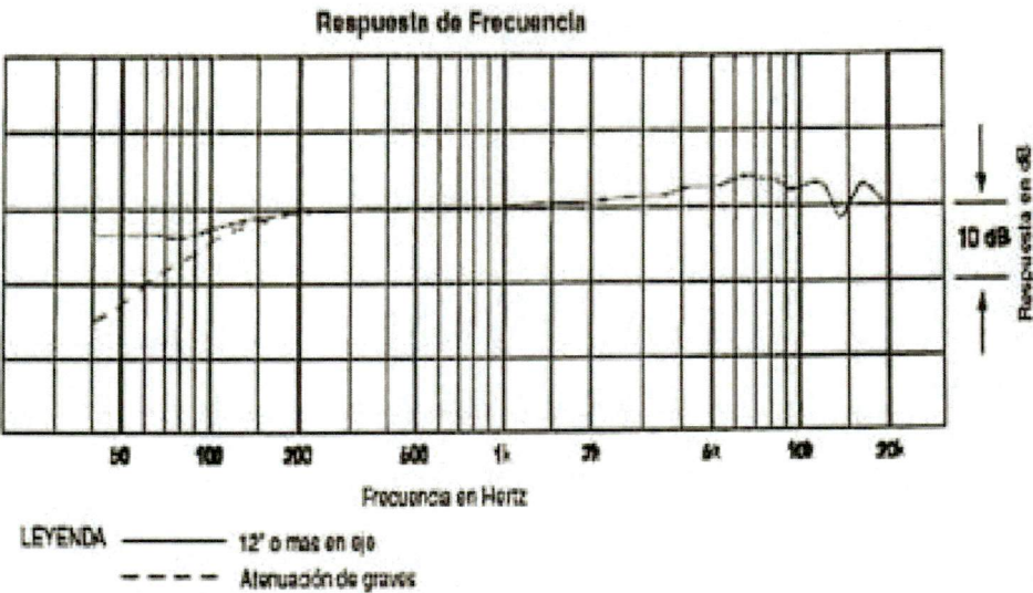
Gráfica 1. Respuesta de Frecuencia del micrófono ATM 450 AUDIO-TECNICA
