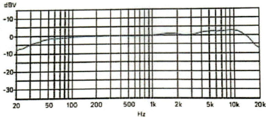
Gráfica 2. Respuesta de Frecuencia del Micrófono SENNHEISER MK4
